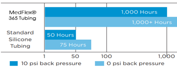
左图 (室温、水介质、零背压) 条件下: 尺寸为 6.4mm*9.5mm 的软管在 600RPM 的三轮蠕动泵驱动下连续不间断工作时长达 1000hrs。
